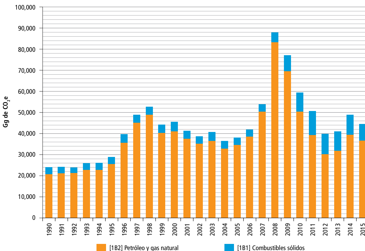
Figura 2.21. Emisiones de GEI por [1B] Emisiones fugitivas provenientes de la fabricación de combustibles, 1990-2015
