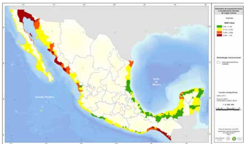
Figura 5.32. Subíndice de exposición a inundaciones litorales de origen marino de los municipios costeros de México, proyectado en el largo plazo
