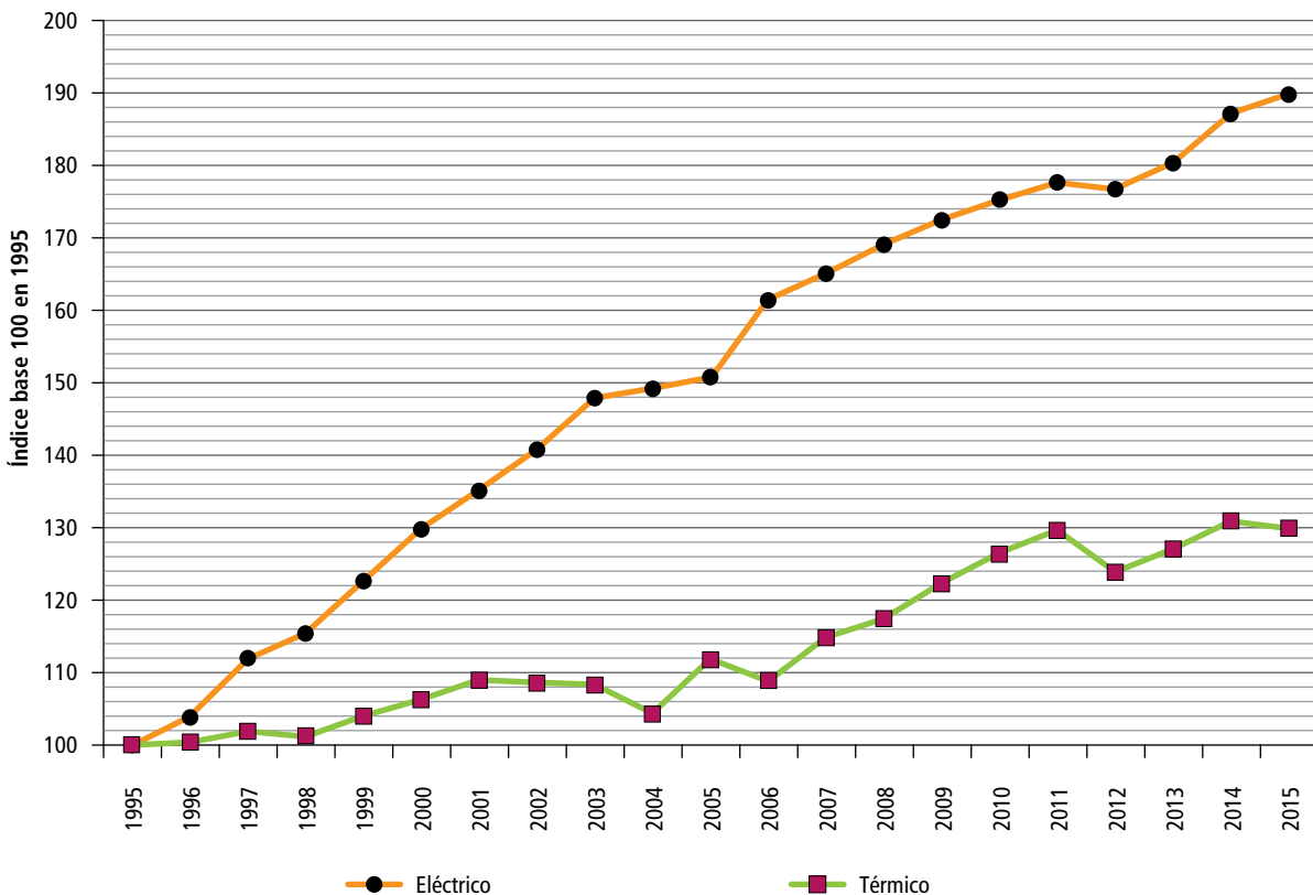
Figura 4.28. Tendencia del crecimiento acumulado del consumo final eléctrico y térmico, 1995-2015
