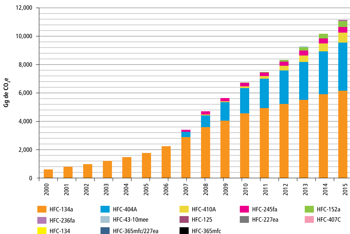
Figura 2.23. Emisiones de hidrofluorocarbonos (HFC)
