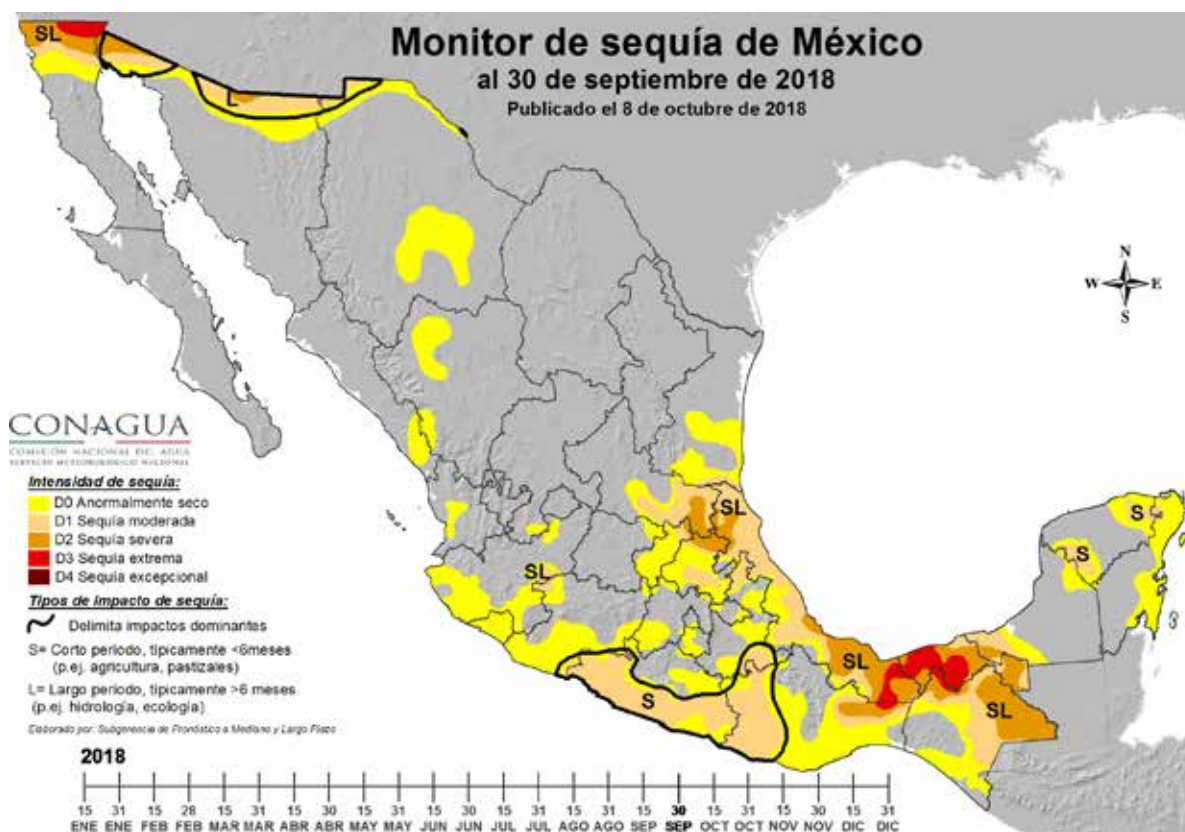
Figura 1.7 Área afectada con sequía en México, septiembre 2018
