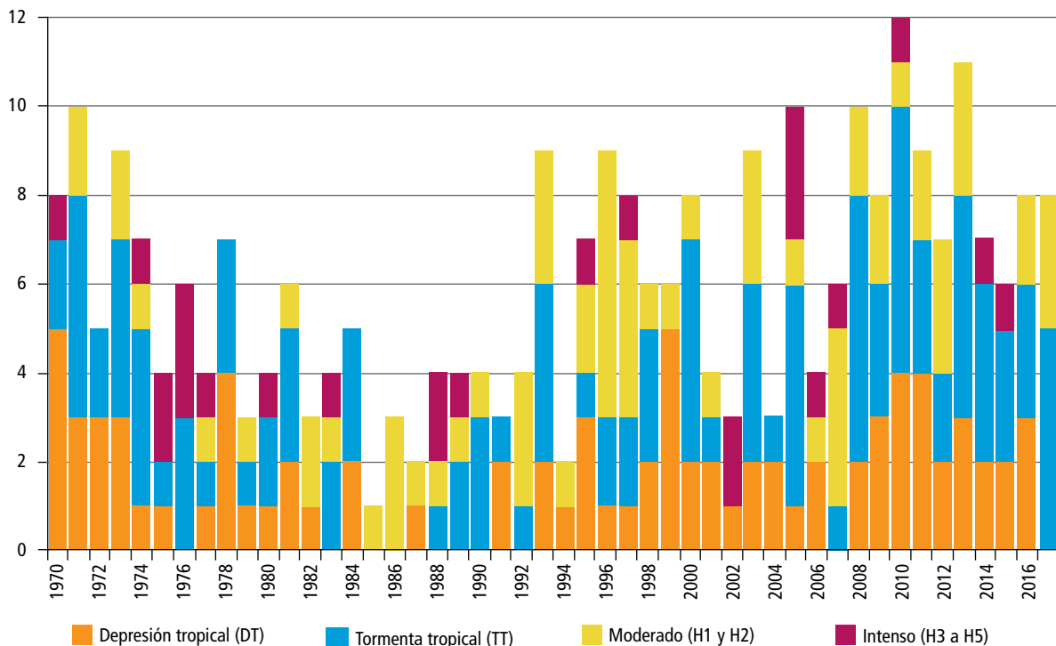
Figura 1.6 Ciclones tropicales que han impactado México, 1970-2017
