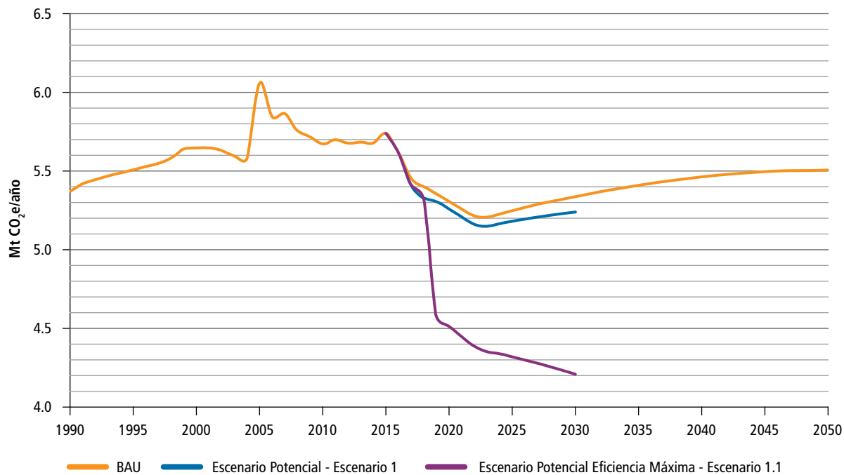
Figura 3.26. Comparación BAU con las emisiones de la medida de mitigación M1
